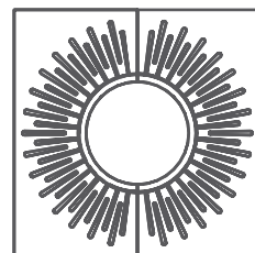
Grille d'Arbre Modèle II Q120 Alcorque Modelo II Q120 01281 120x120x6 cm ≈ 130 kg Encastré Avec Fixation Encastrado con fijación
