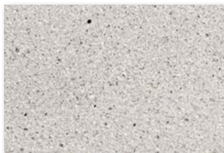
GRANALHADUS GRANITO BEIRÃO MDJ2020411 GRANALHADUS GRANITE BEIRÃO 40x60x2,5 cm / 60x60x2,5 cm ≈ 62 Kg/m 2
