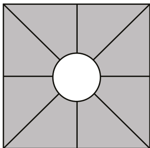
BD1 BASE DUCHA PISCINA BASE DE DOUCHE DE PISCINE Ø 20 / 30 cm 120x120x2,5 cm ≈ 82 kg/Un
